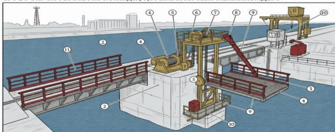
СУРЕТ 3.1: КӨТЕРІЛЕТІН КӨПІРДІҢ ҚҰРЫЛҒЫСЫ МЕН МЕХАНИЗМДЕРІ
